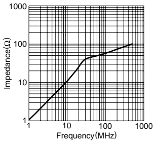
HF57BB3.5X1.5X1.3
